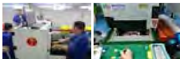
改善前音频测试侧身取放， 手按开关启动
